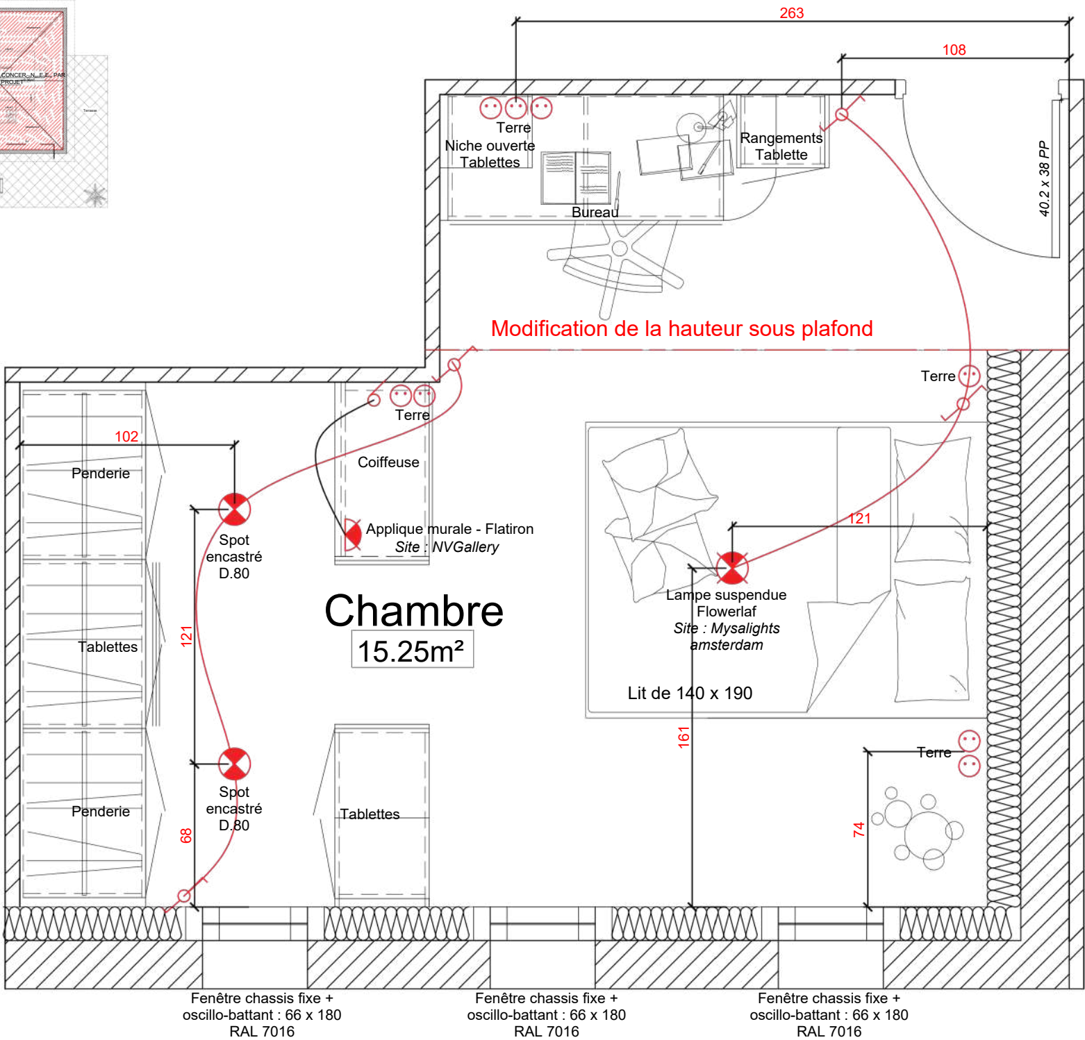
PLAN ELECTRIQUE 1/25
