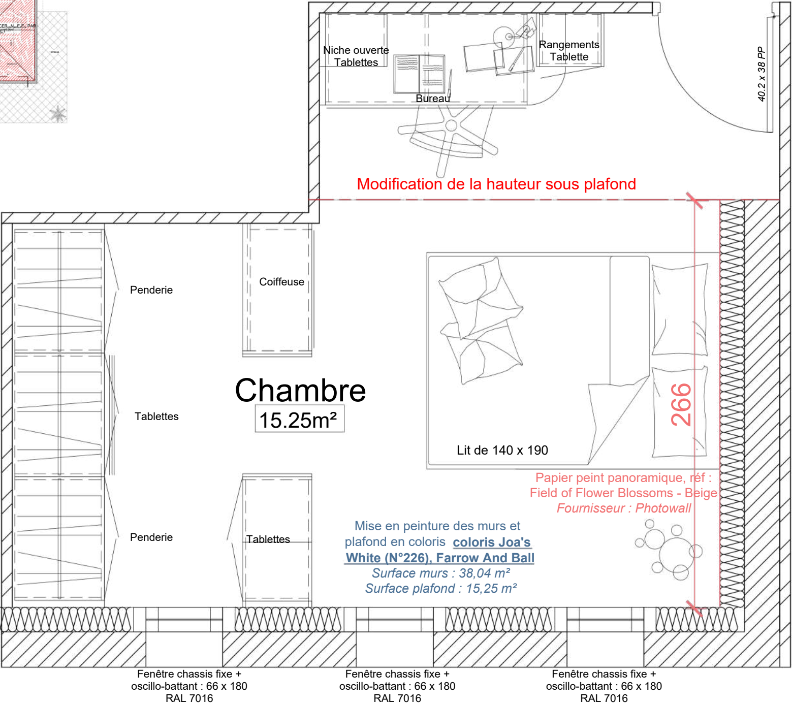
PLAN PEINTURE 1/25
